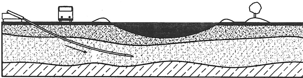
Rys.1) Przewiert pilotażowy
